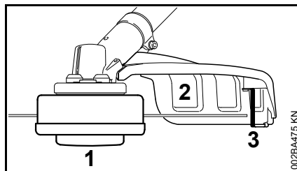
1 Cabeza segadora
